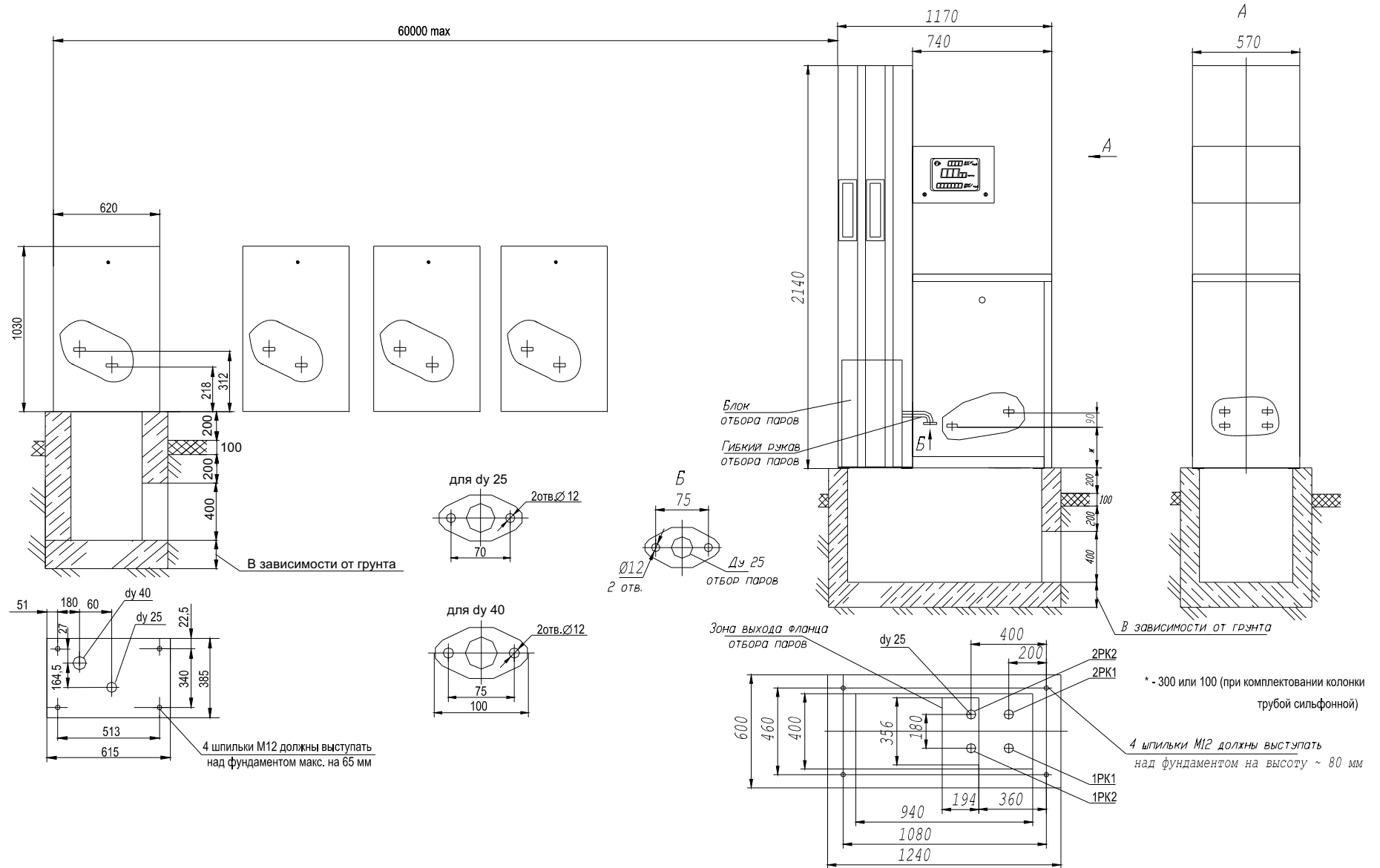
Общий вид колонки на фундаменте.
