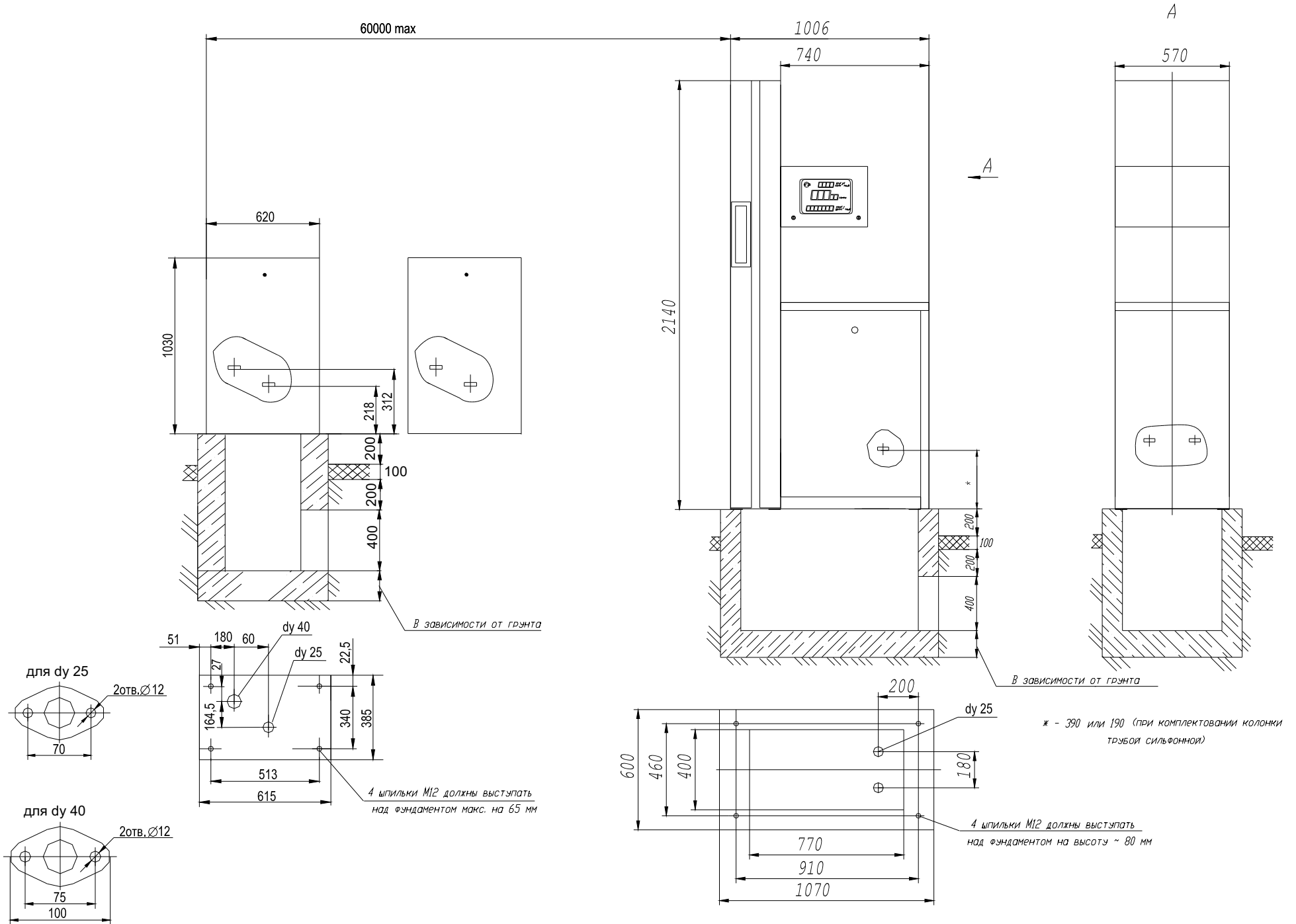
Общий вид колонки на фундаменте.
