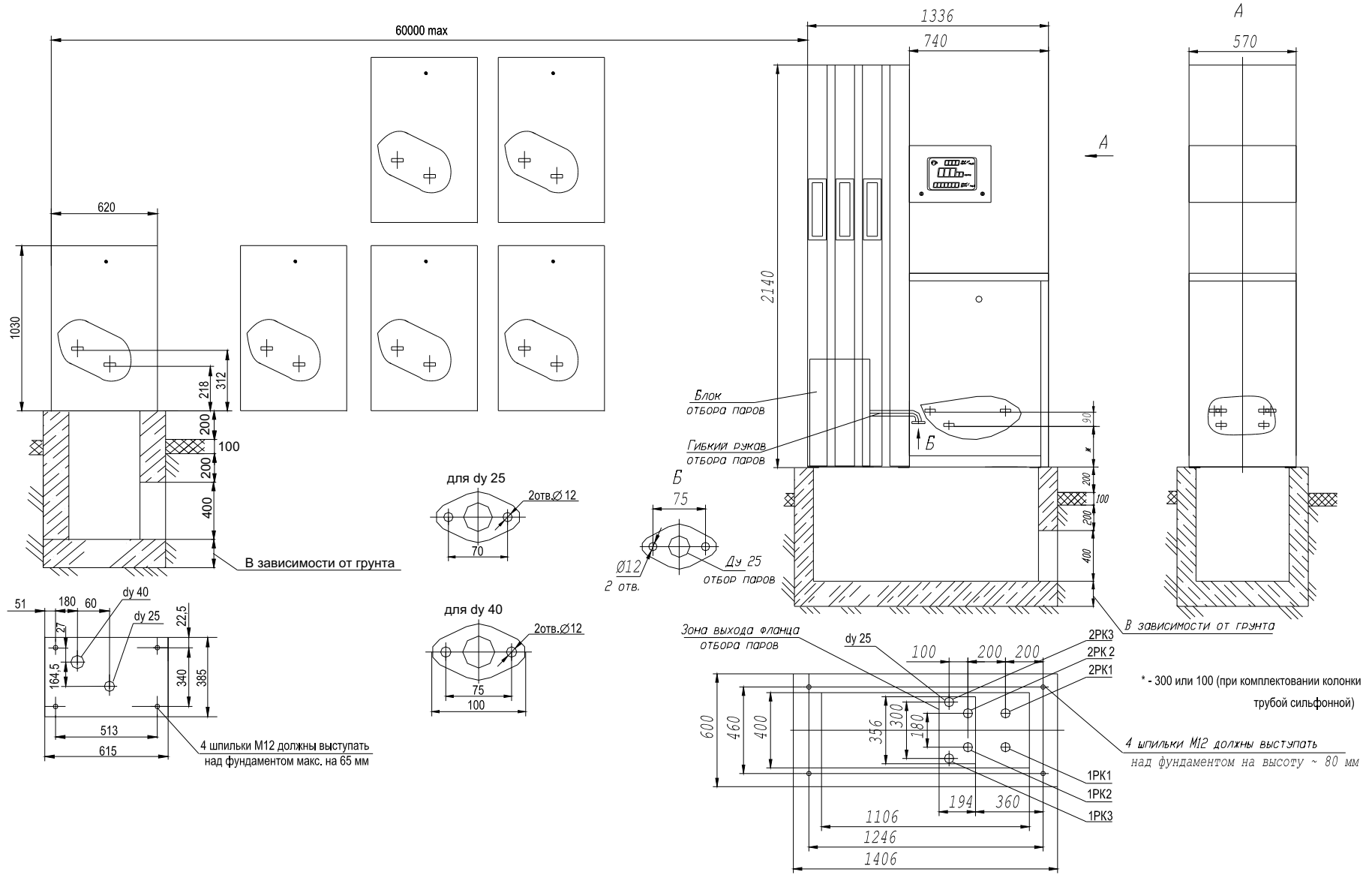
Общий вид колонки на фундаменте.
